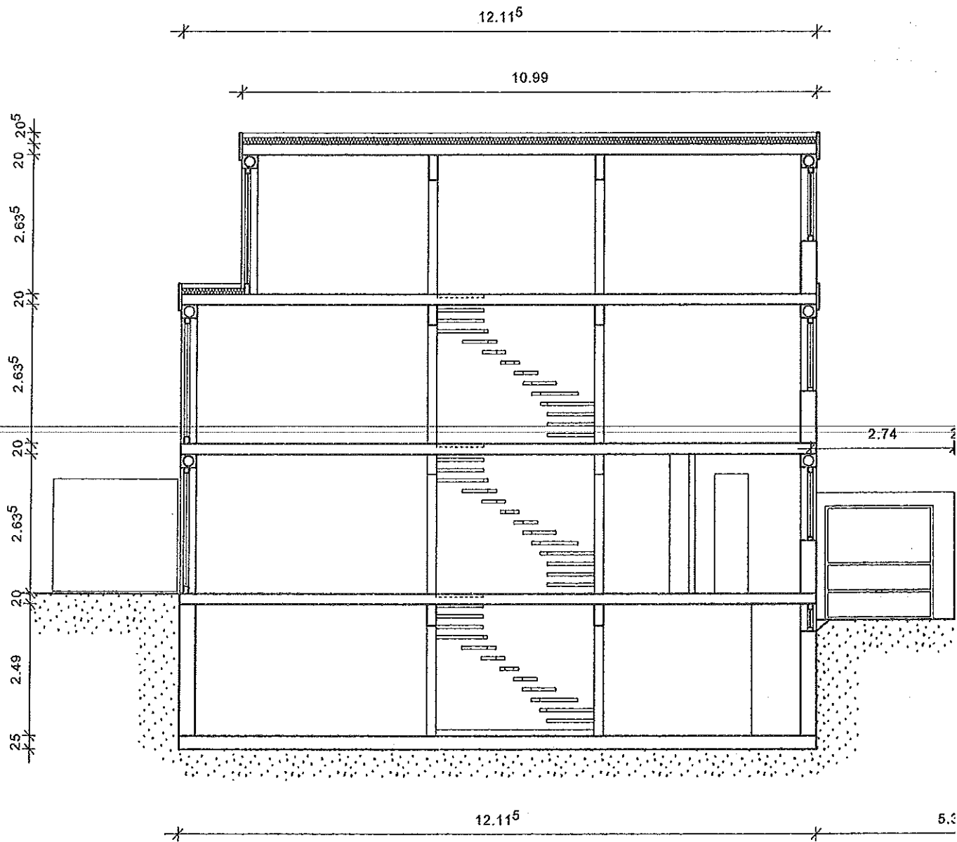
DOPPELHAUS MIT GARAGEN SCHNITT
