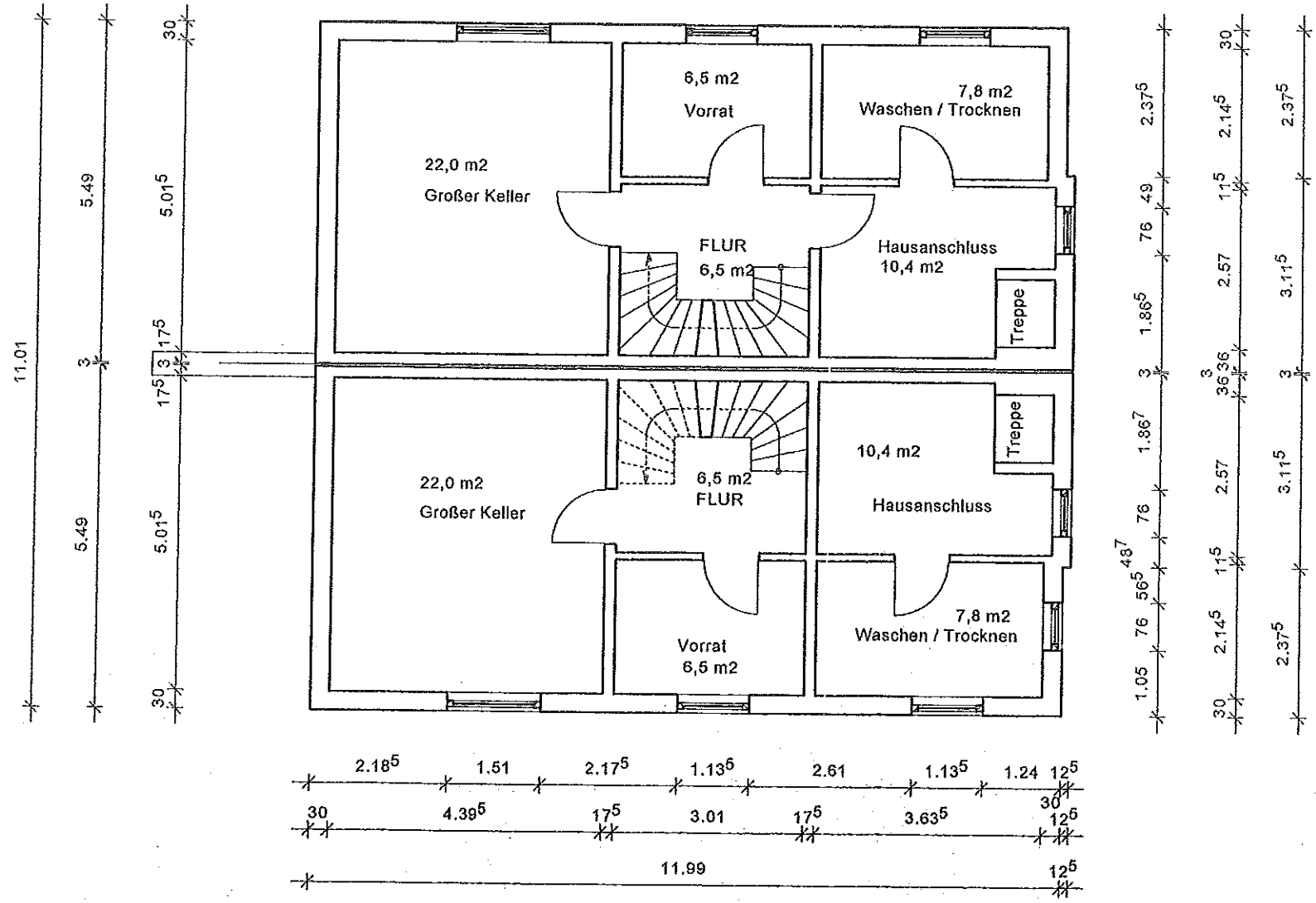
Doppelhaus mit Garagen / Kellergeschoss
